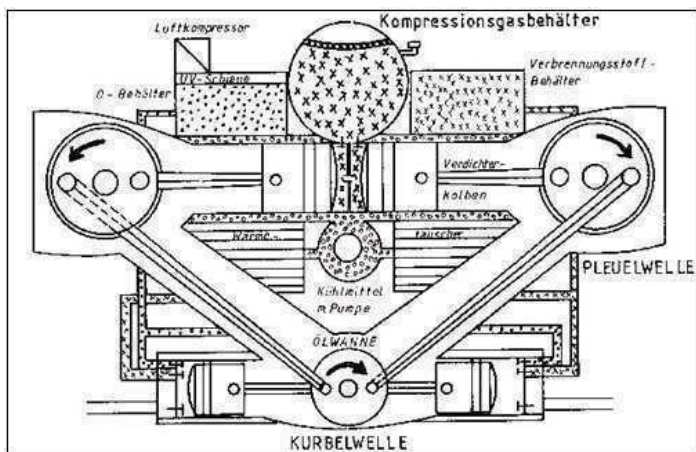
Schema der RLS-Engine
